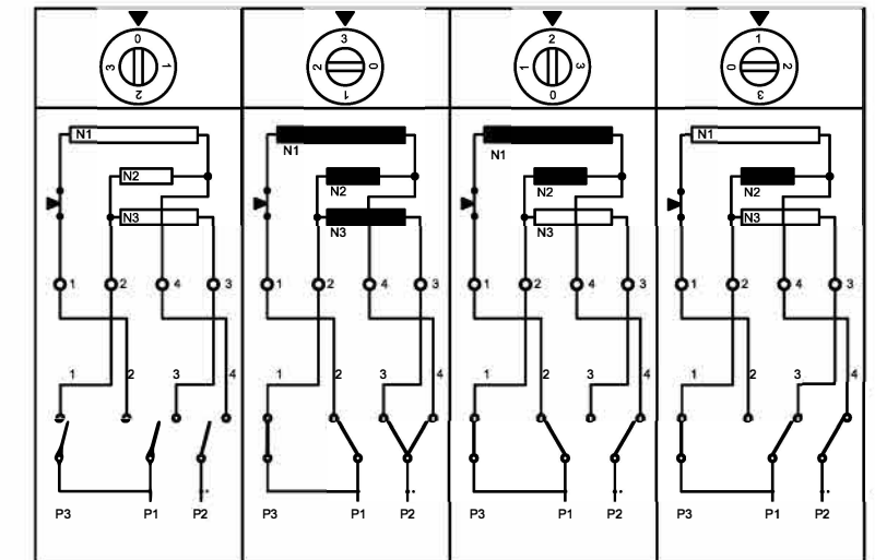
POSICIONES DEL CONMUTADOR DE ESTEATITA.
