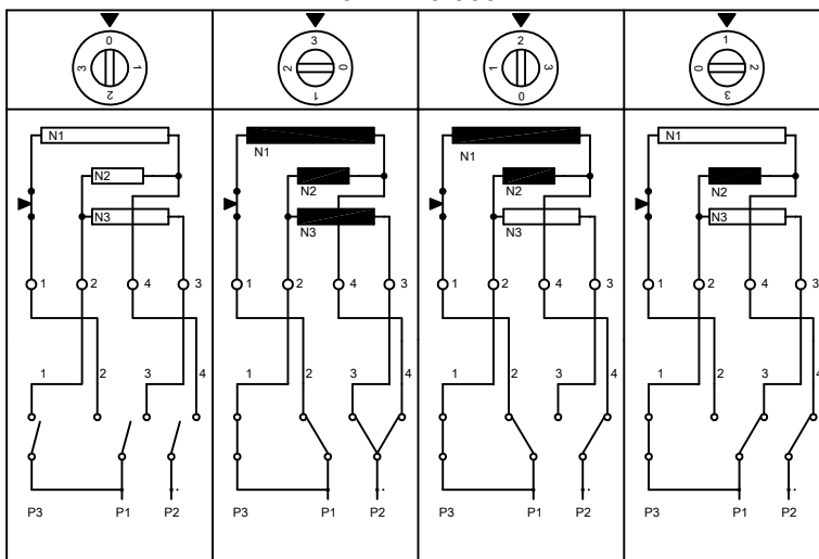
POSICIONES DEL CONMUTADOR DE ESTEATITA. 49.24215.000
